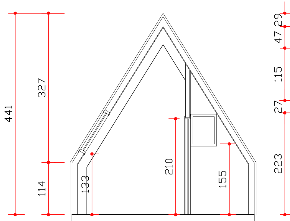
CORTE BB
