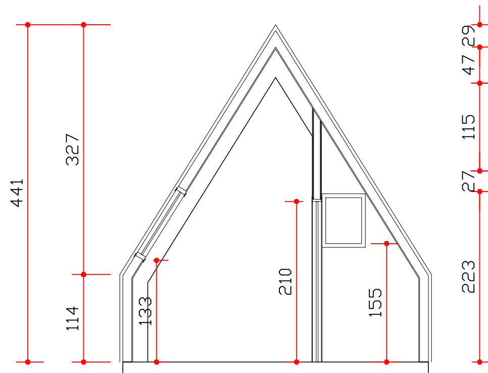
CORTE BB
