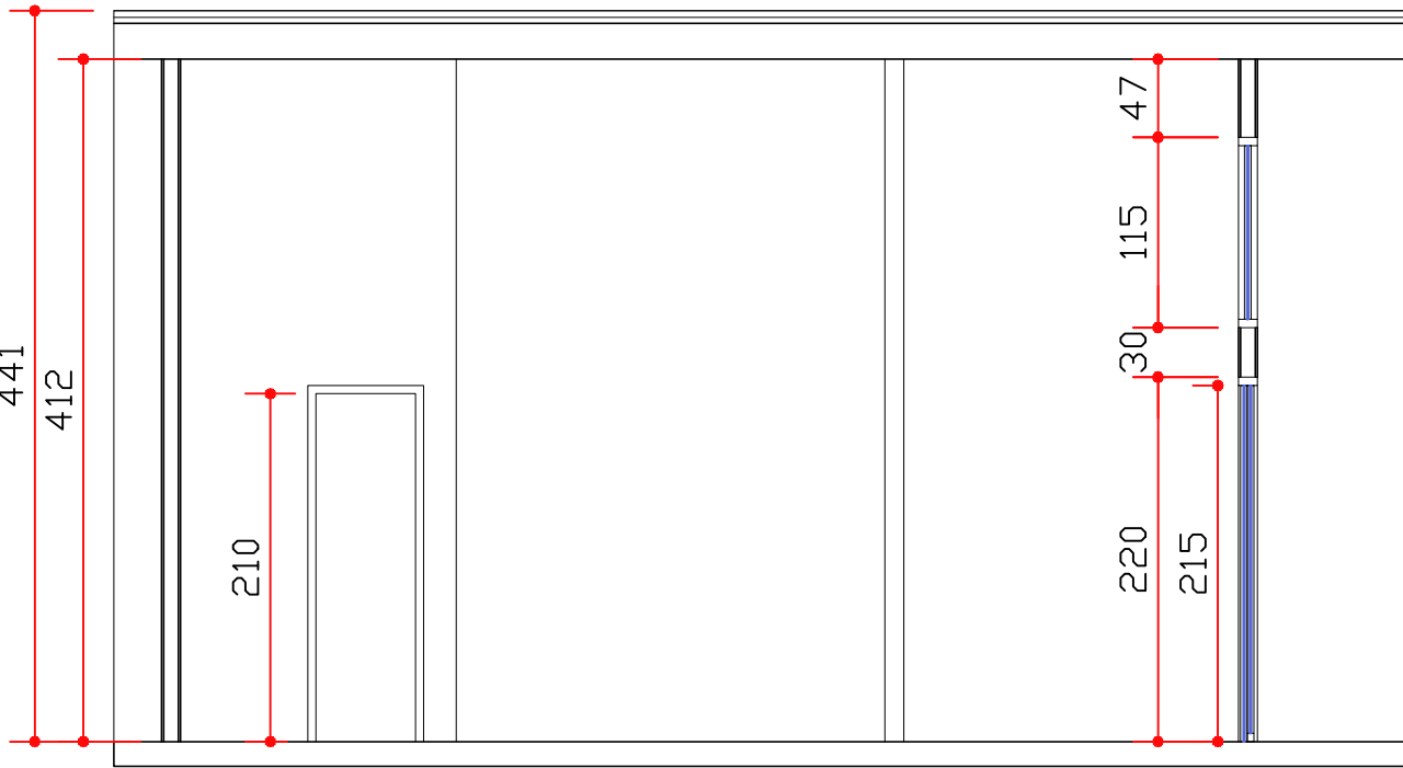
CORTE CC
