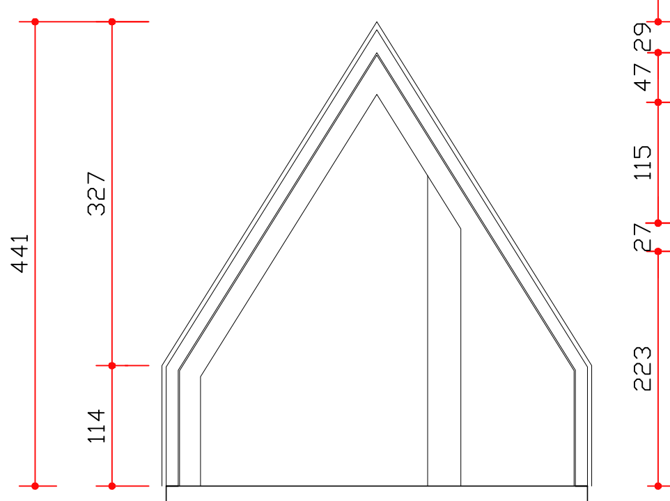
CORTE AA
