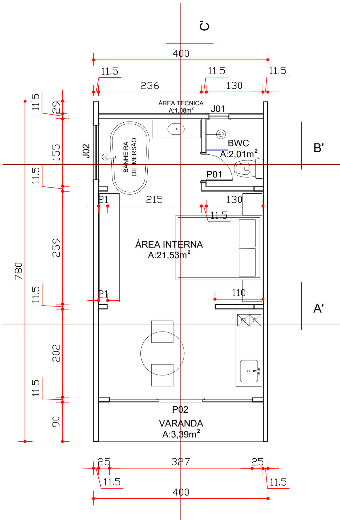
PLANTA BAIXA ESC-1/50
