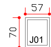
J01 - Maxim ar vão luz 49x59cm
