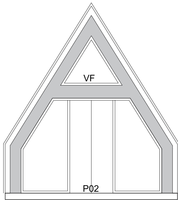
ELEVAÇÃO FRONTAL
